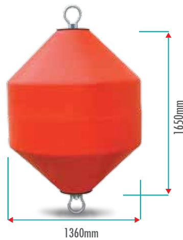
M03290 1600 LT ŞAMANDIRA / BUOY Yüzdürmesi / Buoyancy: 1500 kg Ürün Ağırlığı / Weight: 110 kg
