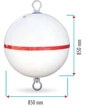
M03325 320 LT ŞAMANDIRA / BUOY Yüzdürmesi / Buoyancy: 290 kg Ürün Ağırlığı / Weight: 30 kg
