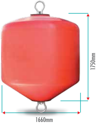
M03280 2500 LT ŞAMANDIRA / BUOY Yüzdürmesi / Buoyancy: 2250 kg Ürün Ağırlığı / Weight: 166 kg
