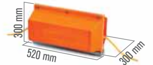
M03518 26 LT Ağırlık / Weight : 4,5 kg Yüzdürme / Buoyancy : 23 kg
