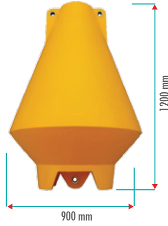
M03326 350 LT ŞAMANDIRA / BUOY Yüzdürmesi / Buoyancy: 295 kg Ürün Ağırlığı / Weight: 80 kg
