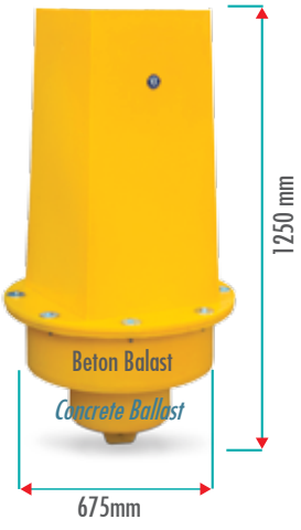
M03255 180 LT ŞAMANDIRA / BUOY Ürün Ağırlığı / Weight: 18 kg
