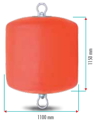
M03300 1200 LT ŞAMANDIRA / BUOY Yüzdürmesi / Buoyancy: 1000 kg Ürün Ağırlığı / Weight: 90 kg
