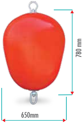
M03091 170 LT ŞAMANDIRA / BUOY Yüzdürmesi / Buoyancy: 155 kg Ürün Ağırlığı / Weight: 18 kg
