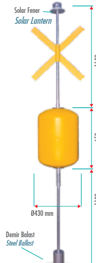
M03260 26 kg ŞAMANDIRA / BUOY
