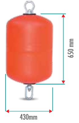
M03350 100 LT ŞAMANDIRA / BUOY Yüzdürmesi / Buoyancy: 90 kg Ürün Ağırlığı / Weight: 11 kg
