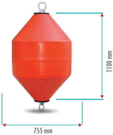
M03330 300 LT ŞAMANDIRA / BUOY Yüzdürmesi / Buoyancy: 250 kg Ürün Ağırlığı / Weight: 28 kg
