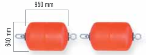
M03524 200 LT Ağırlık / Weight : 22 kg Yüzdürme / Buoyancy : 180 kg
